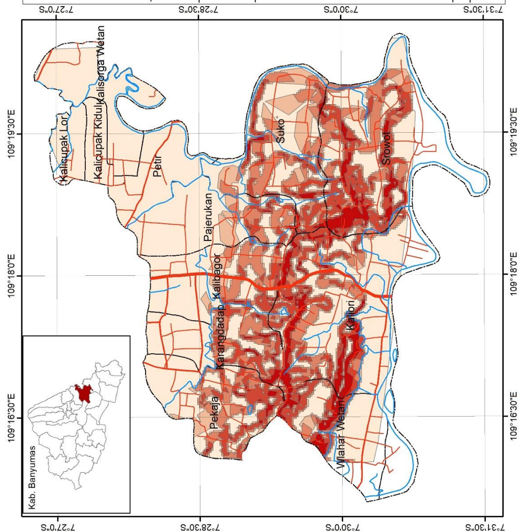
Lampiran 25 Peta Kelas Lereng Kecamatan Kalibagor
